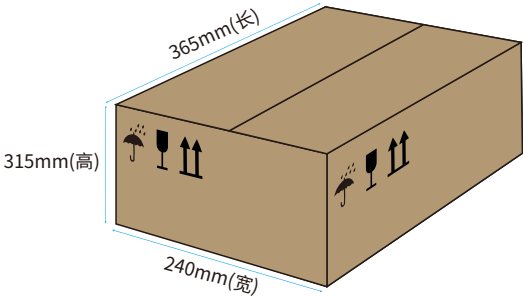
(外箱尺寸)
