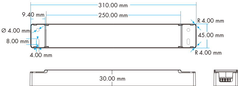
(产品尺寸)
