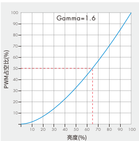
对数调光曲线
