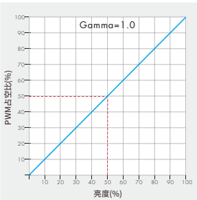
线性调光曲线
