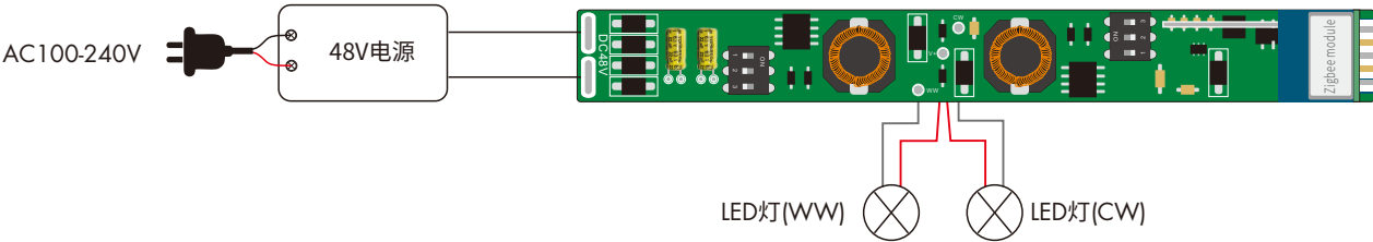
系统接线图
