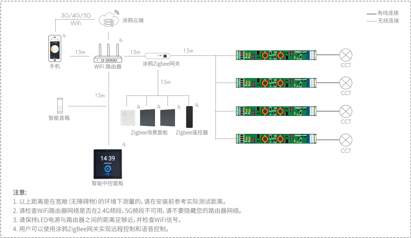
系统接线图
