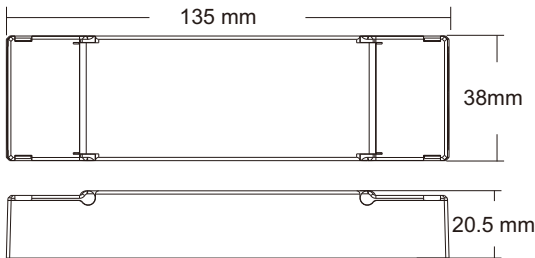
(产品尺寸)
